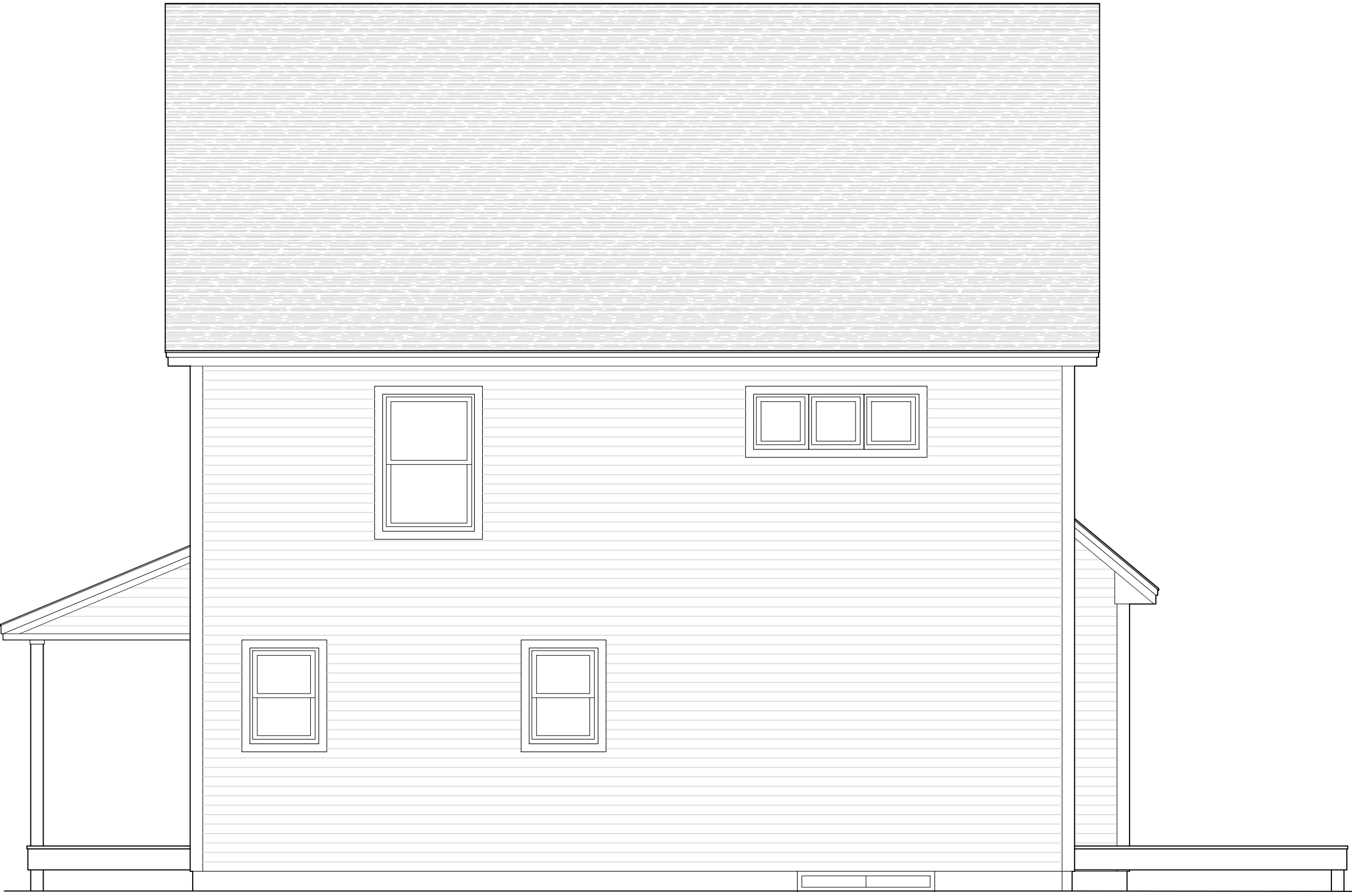
Right Elevation
